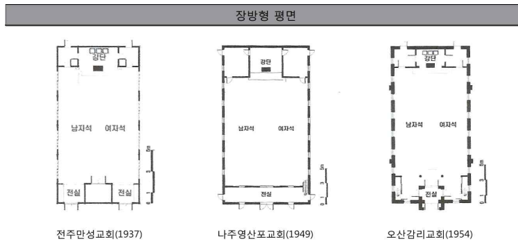
<그림-15> 장방형 평면 사례
