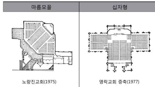
<그림-19> 1970년대 평면유형(2)
